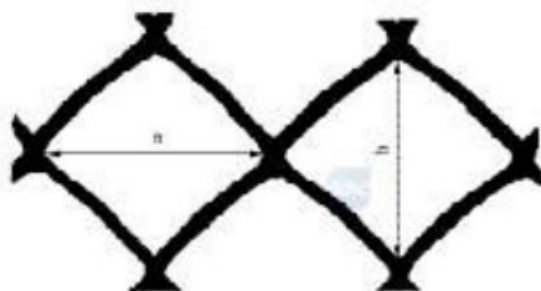
图 6 CE151 网孔测量部位
