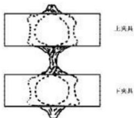
图 10 CE131 纵向试样
